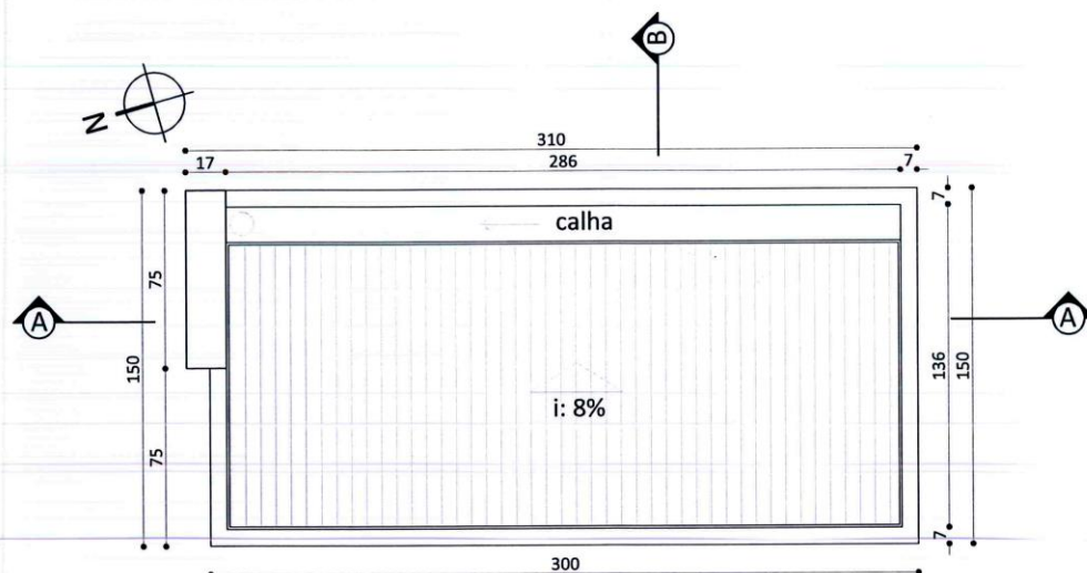
PLANTA COBERTURA Esc.: 1/25
