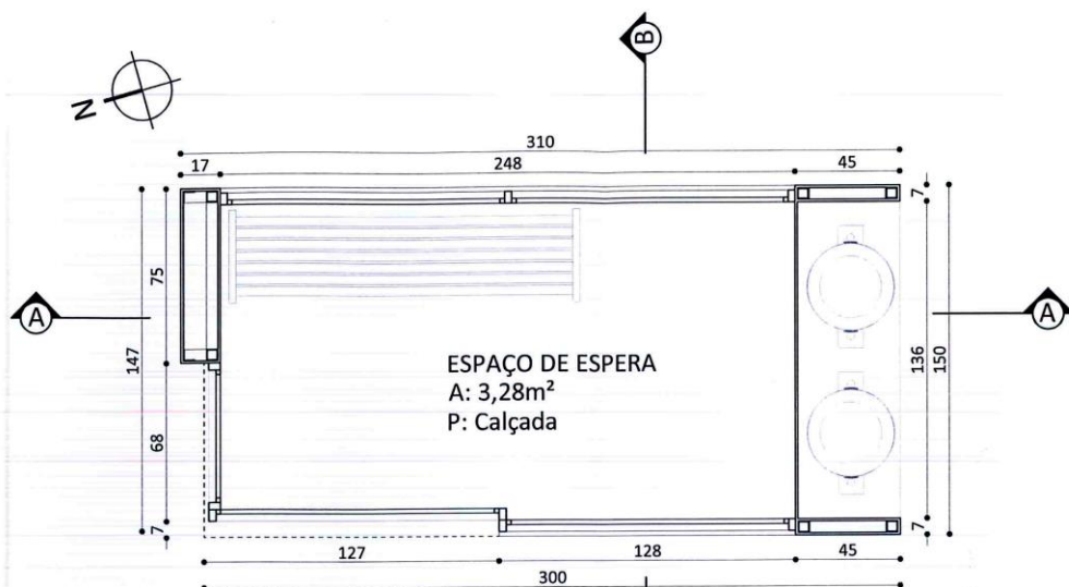
PLANTA BAIXA TÉRREA Esc.: 1/25
